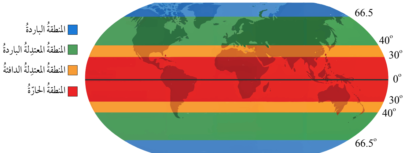
الشكل (1): المناطق الحرارية الرئيسية في العالم.
