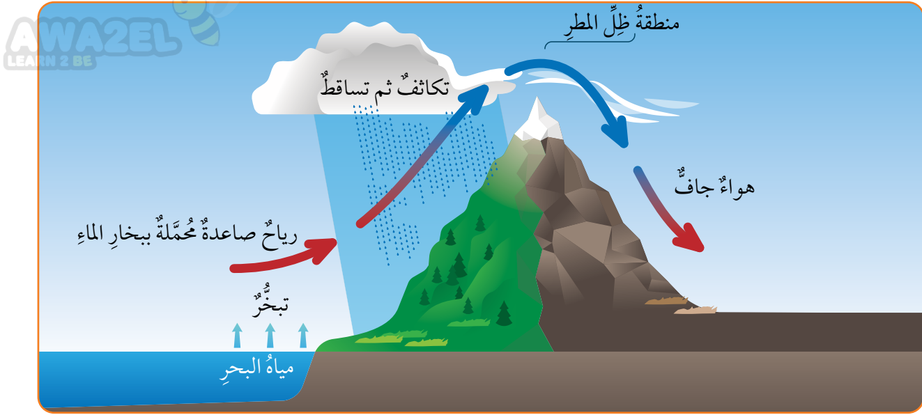
الشكل (8): كيفية حدوث الأمطار التضاريسية.
