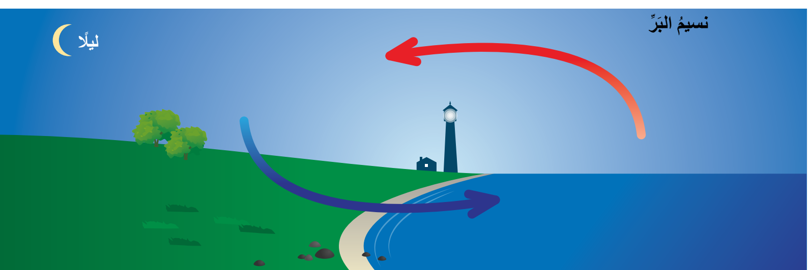
الشكل (6): آلية حدوثِ نسيم البرِّ ونسيم البحرِ.
